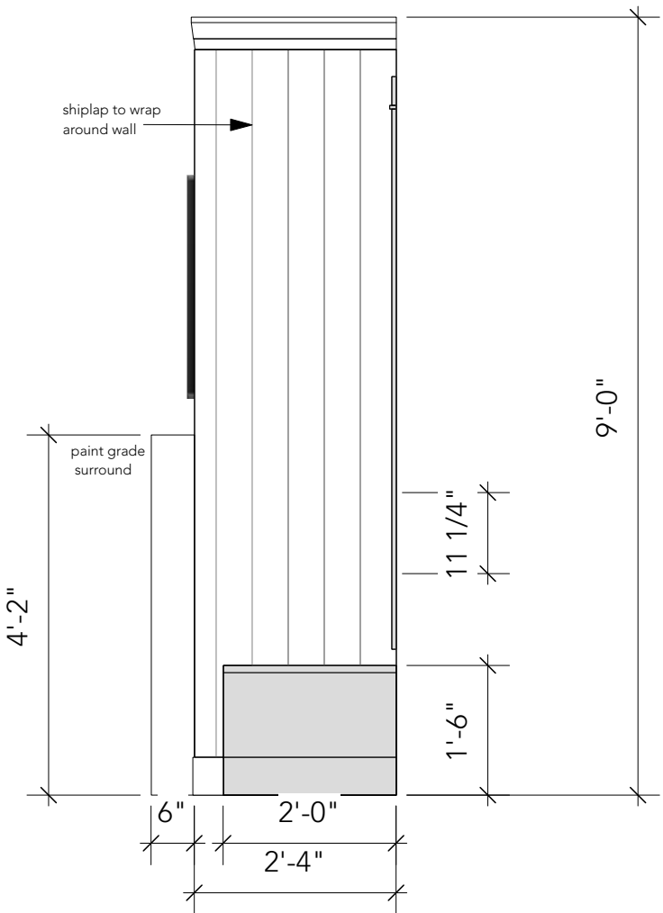
SIDE VIEW SCALE: 1/2" = 1'-0"
