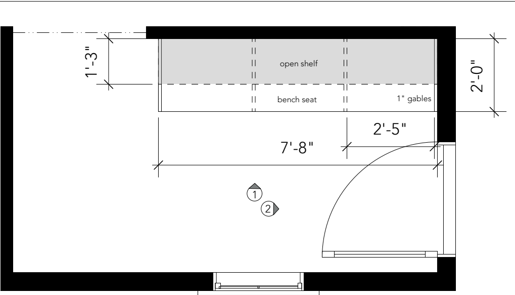
MUDROOM PLAN SCALE: 3/8" = 1'-0"
