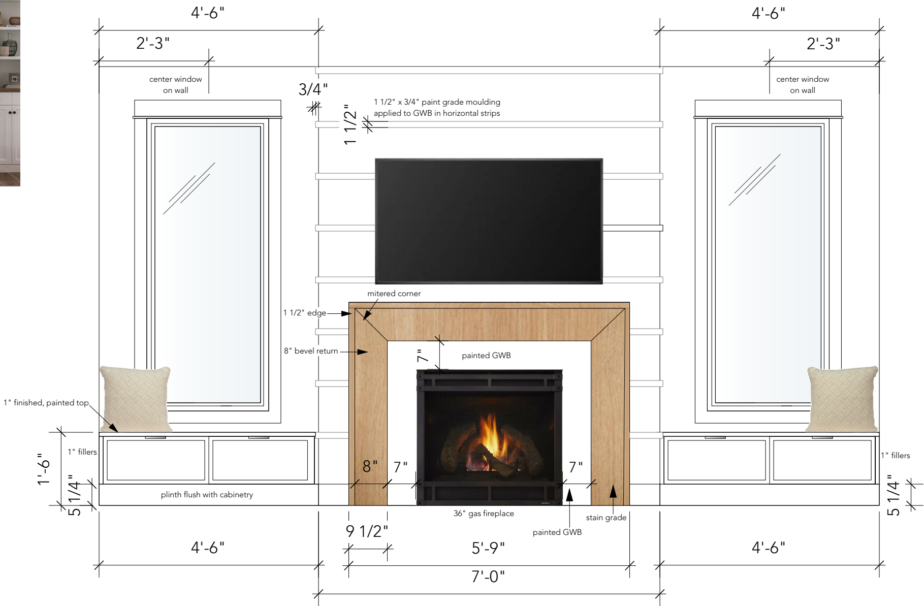
FRONT ELEVATION SCALE: 1/2" = 1'-0"
