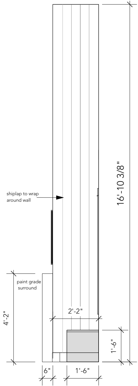
SIDE VIEW SCALE: 3/8" = 1'-0"
