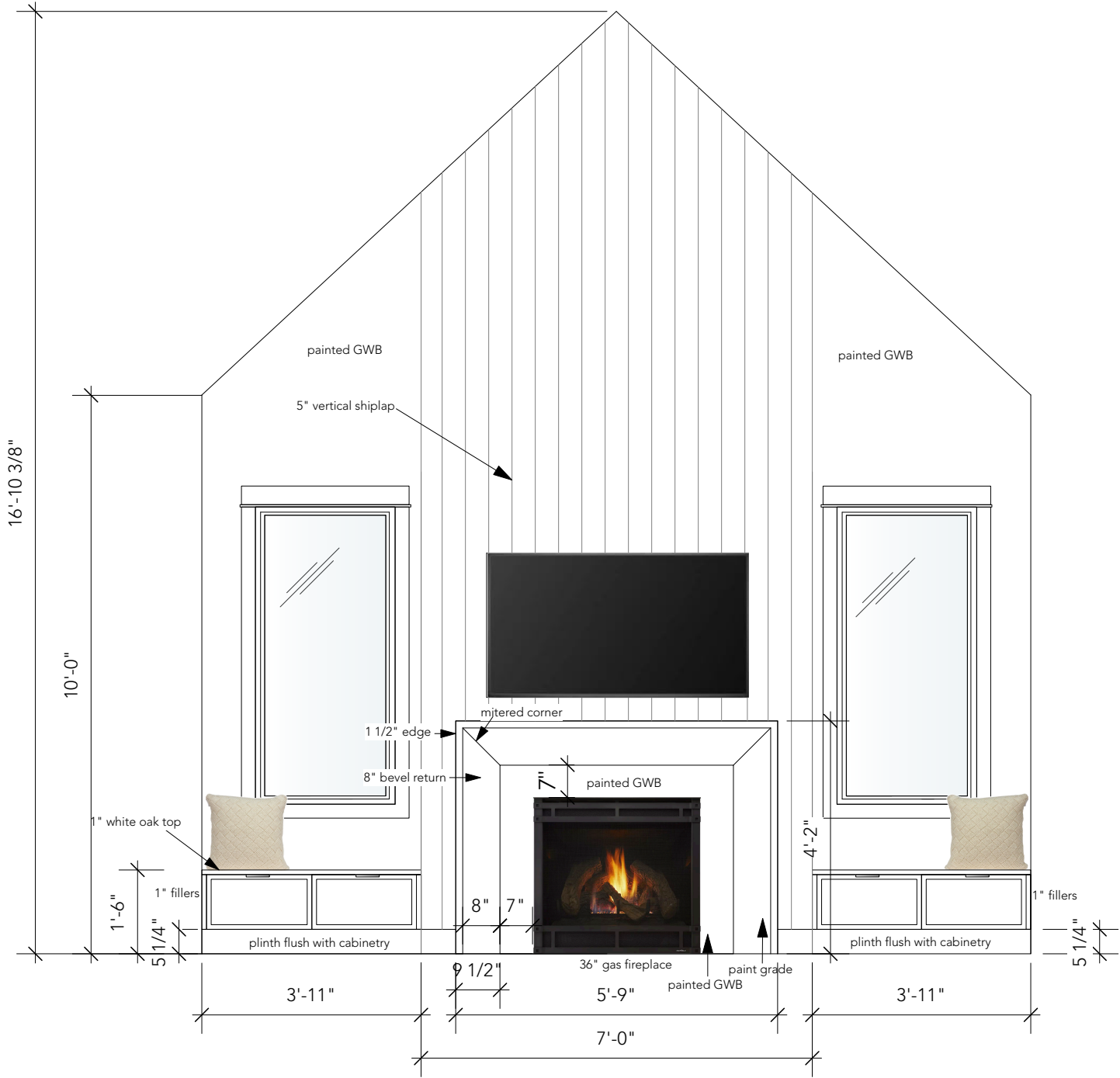
FRONT ELEVATION SCALE: 3/8" = 1'-0"
