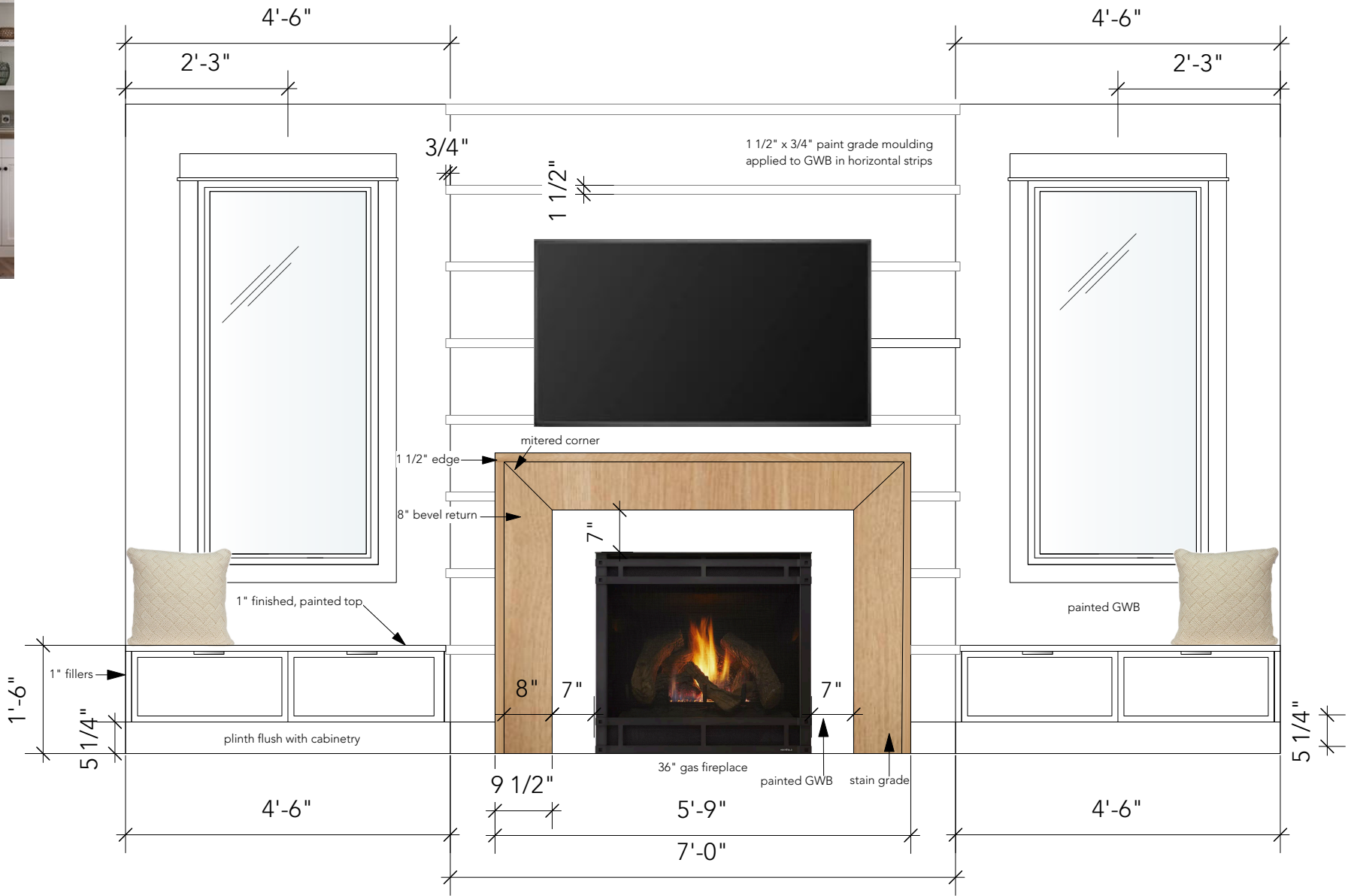
FRONT ELEVATION SCALE: 1/2" = 1'-0"
